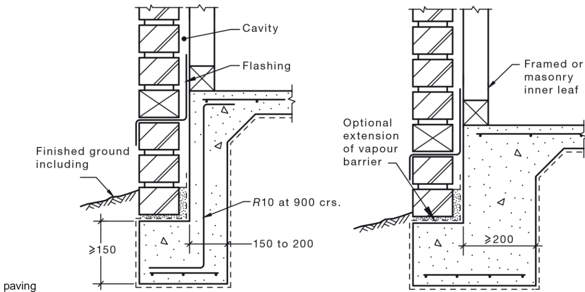
(b) Deep edge rebate alternative
